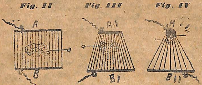
Fig. N. II.—Electrodios iguaes e parallelos, calor maximo equidistante dos dois, em a.
